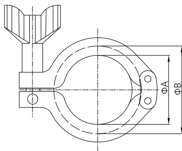
ISO1127 双销式
