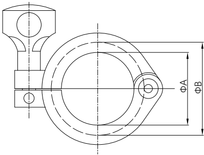
ISO1127 单销式
