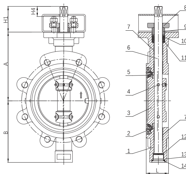
Fig.3645 Lug Type
